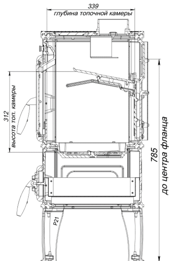
A-A (1 : 7)
