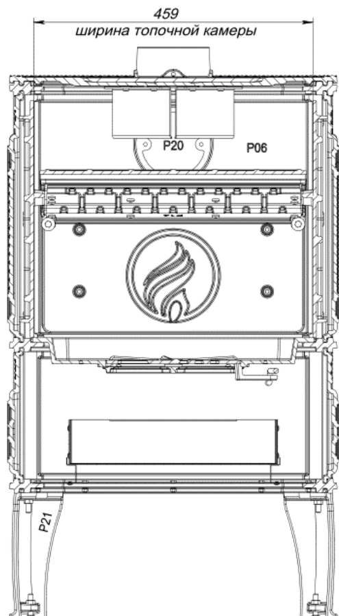
Б-Б (1 : 7)
